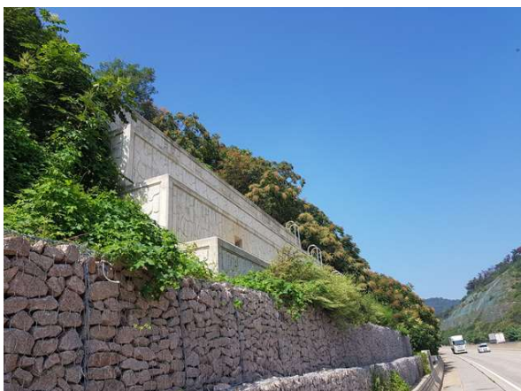
옹벽, 개비온 전경
